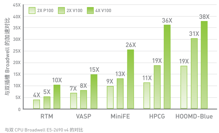
常用 HPC 应用程序配备 Tesla V100 后运行速度更快
