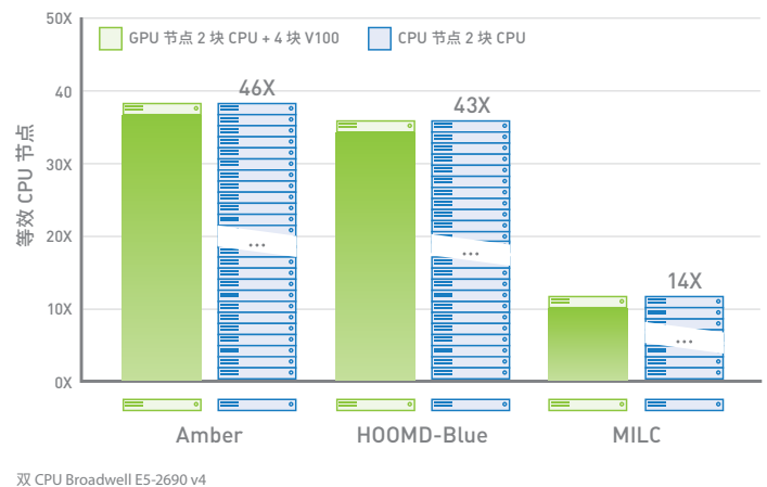
单个 GPU 节点的卓越性能
